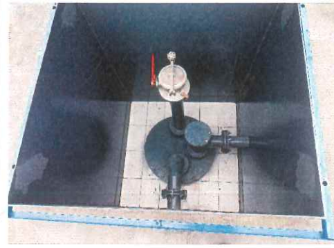
量油口
