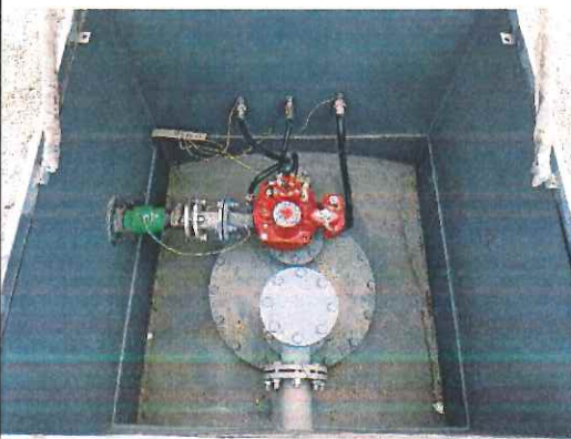
操作井
