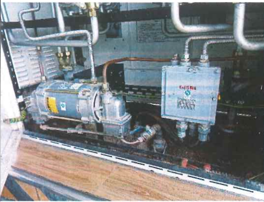
加油机内部
