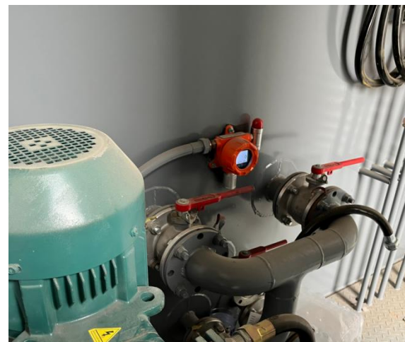
可燃气体检测探头
