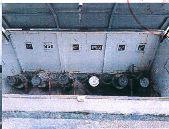
卸油口
