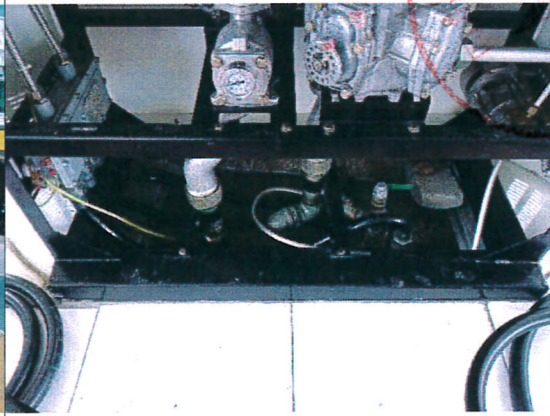
加油机内部
