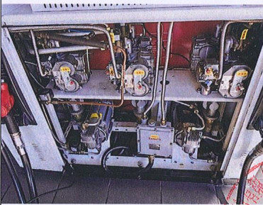
加油机内部
