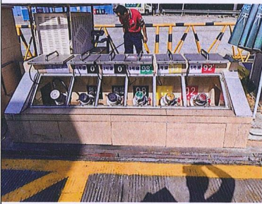
卸油口
