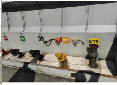
卸油口
