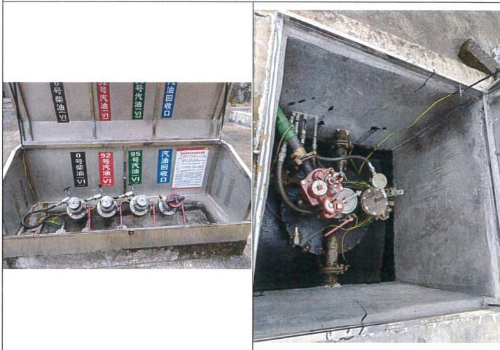
卸油口
