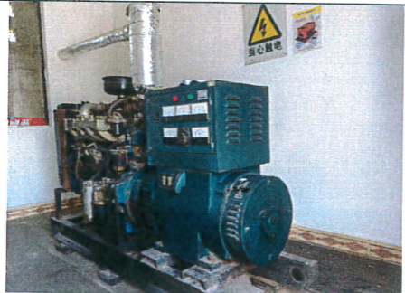
发电机
