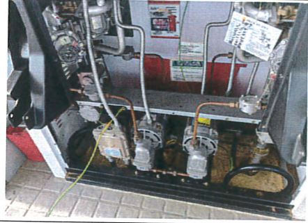
加油机内部
