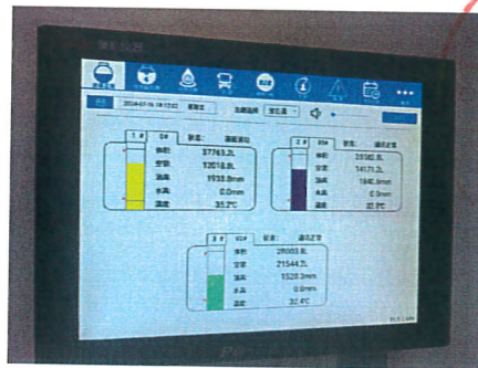
液位计
