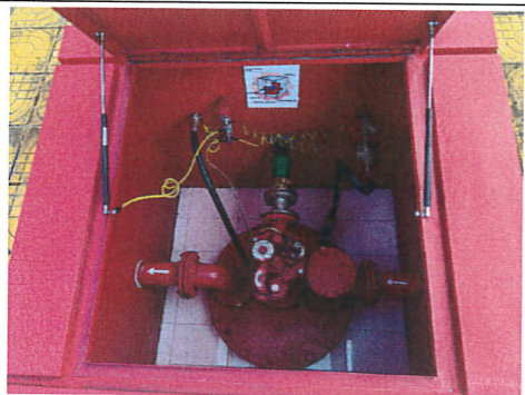
储罐操作井
