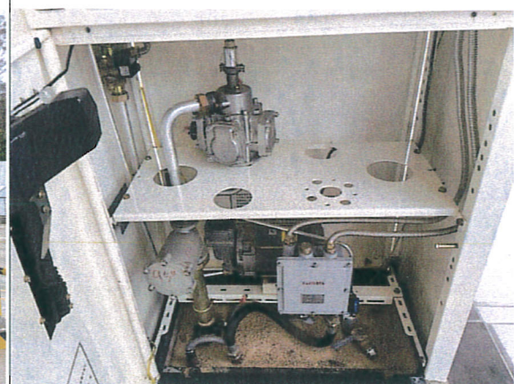
加油机内部
