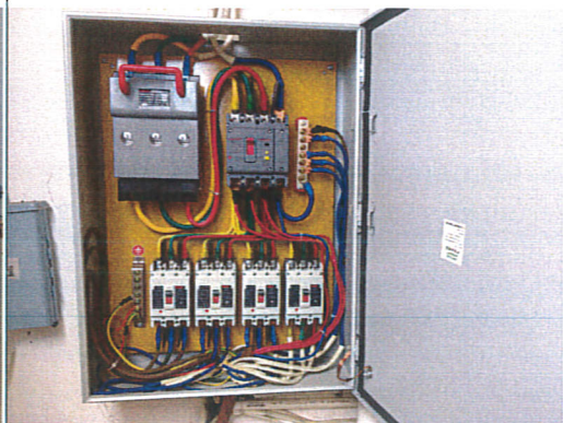
配电箱
