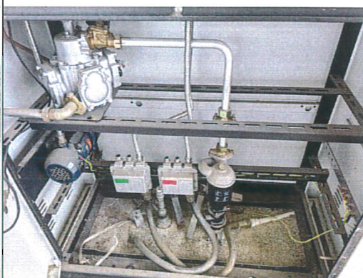
加油机内部
