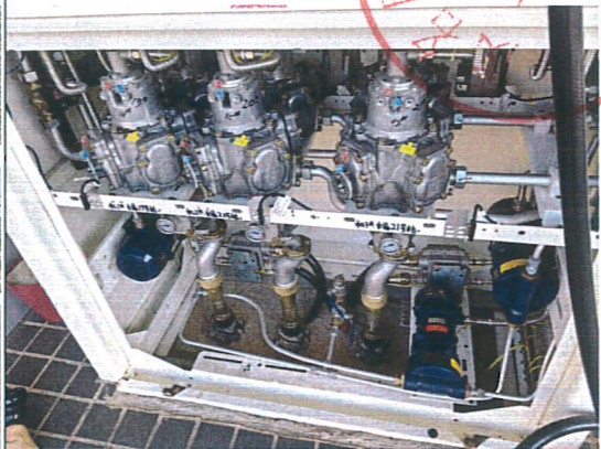
加油机内部
