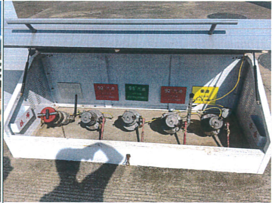
卸油口
