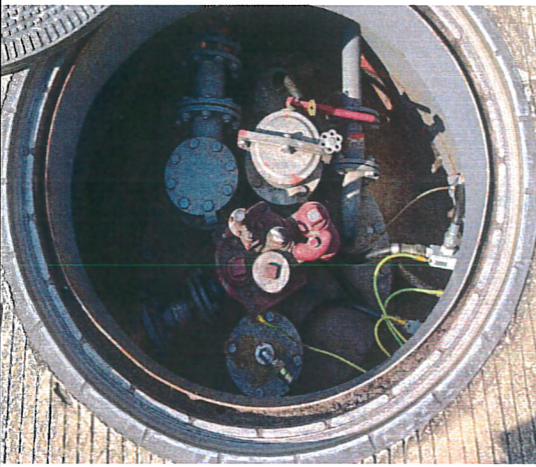
储罐操作井
