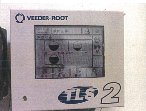
液位计
