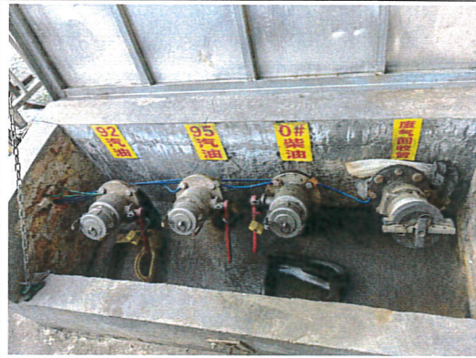
卸油口
