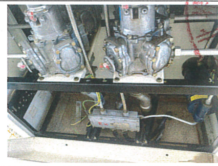
加油机内部
