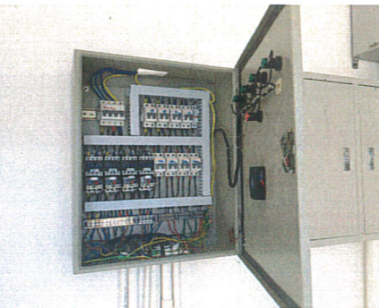
配电柜
