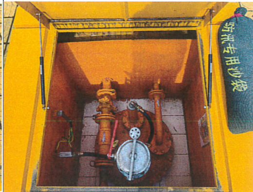
储罐操作井
