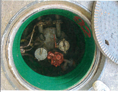
储罐操作井
